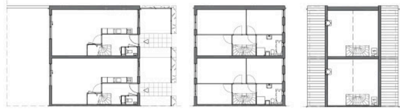
woningen met zadeldak, begane grond / eerste verdieping / tweede verdieping
